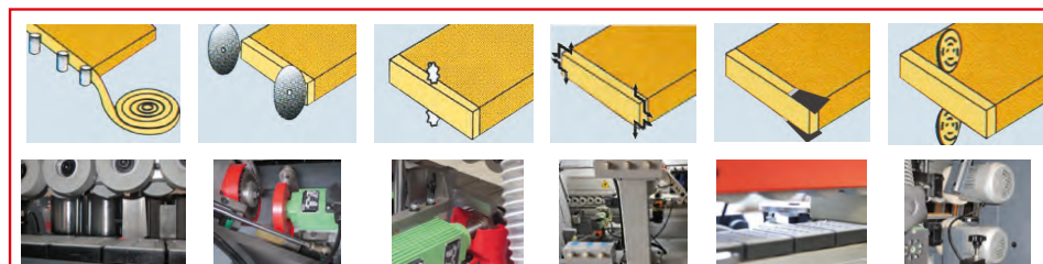
Kleben glueing
