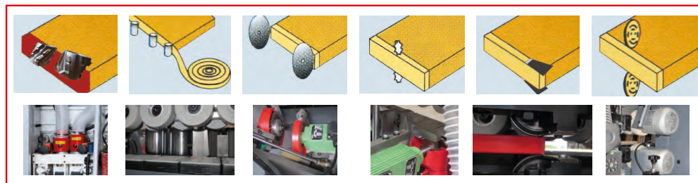
Vorfräser pre-milling
