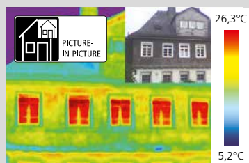
Beeld-in-beeld: infrarood/digitaal beeld
