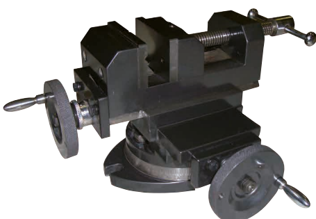
SK 85 Schraubstock-Kreuztisch Kombi- nation / compound slide vice
