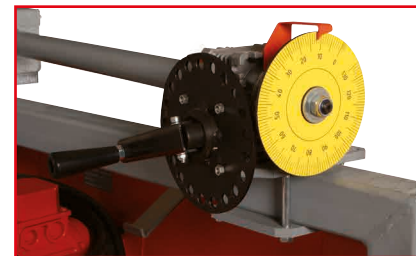
Höhenverstellung des Sägeaggregats erfolgt über Handrad mit Skala height adjustment of saw unit via hand wheel with scale
