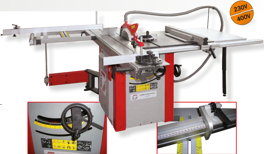
Sägeblatthöhenverstellung saw blade height adjustment
