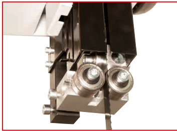
10-fach kugelgelagerte Sägebandführung multiple (10pcs) ball bearing saw band guide
