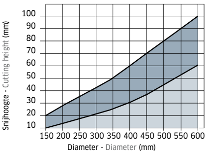
Maximale diepte langs en dwars op basis van de blad-diameter.
