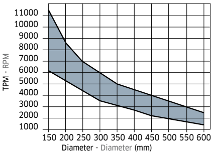
Minimaal en maximaal toerental op basis van blad-diameter.
