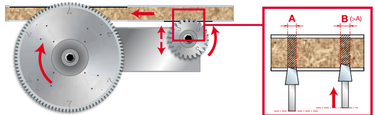
Snijvoeg van hoofdzaagblad Cutting kerf of main saw blade
